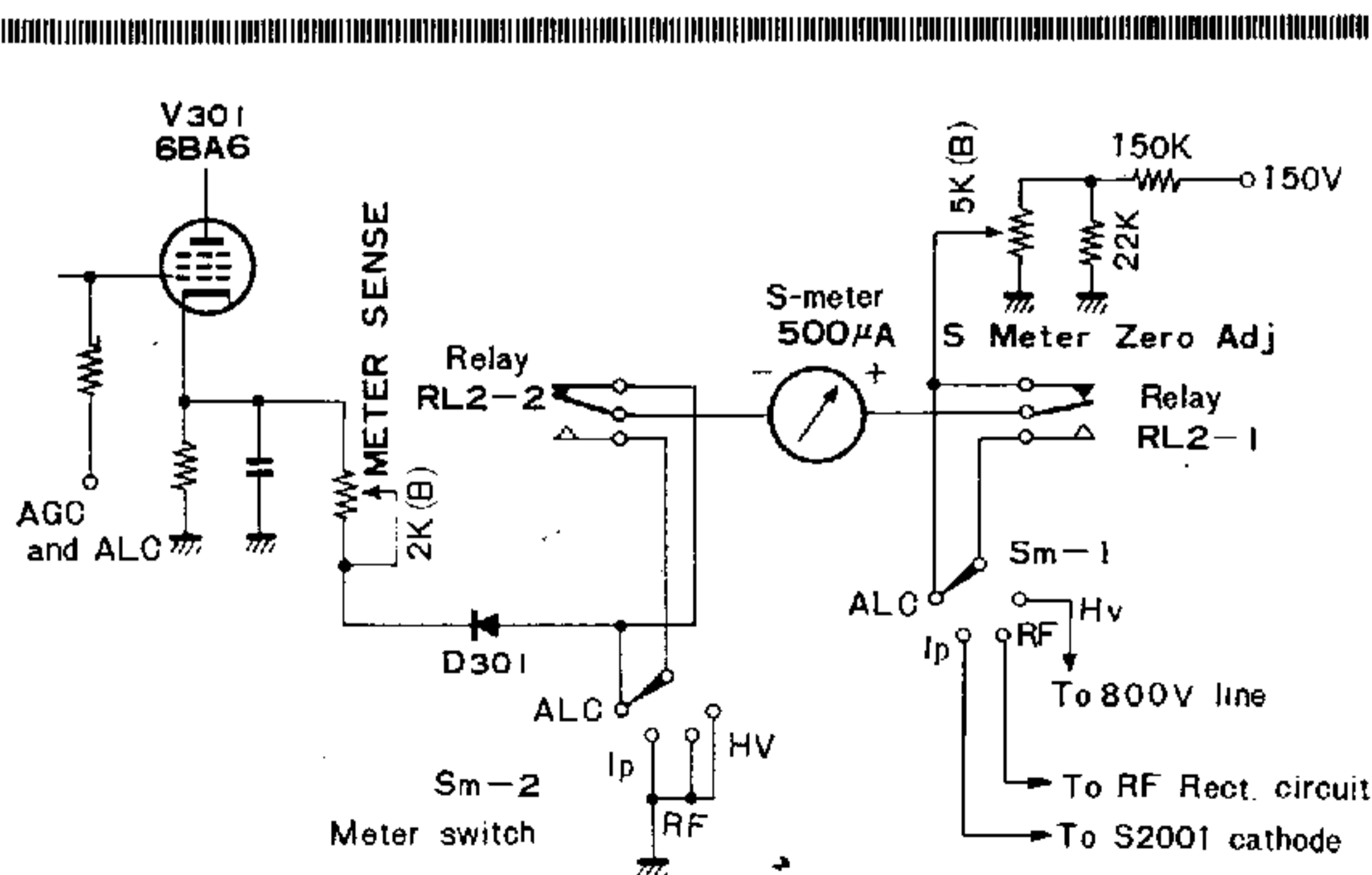
Fig. 9 Meter circuit
