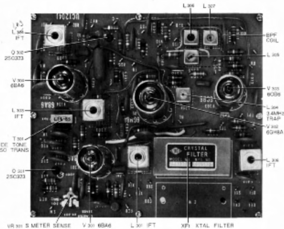
Fig. 22 IF Block
